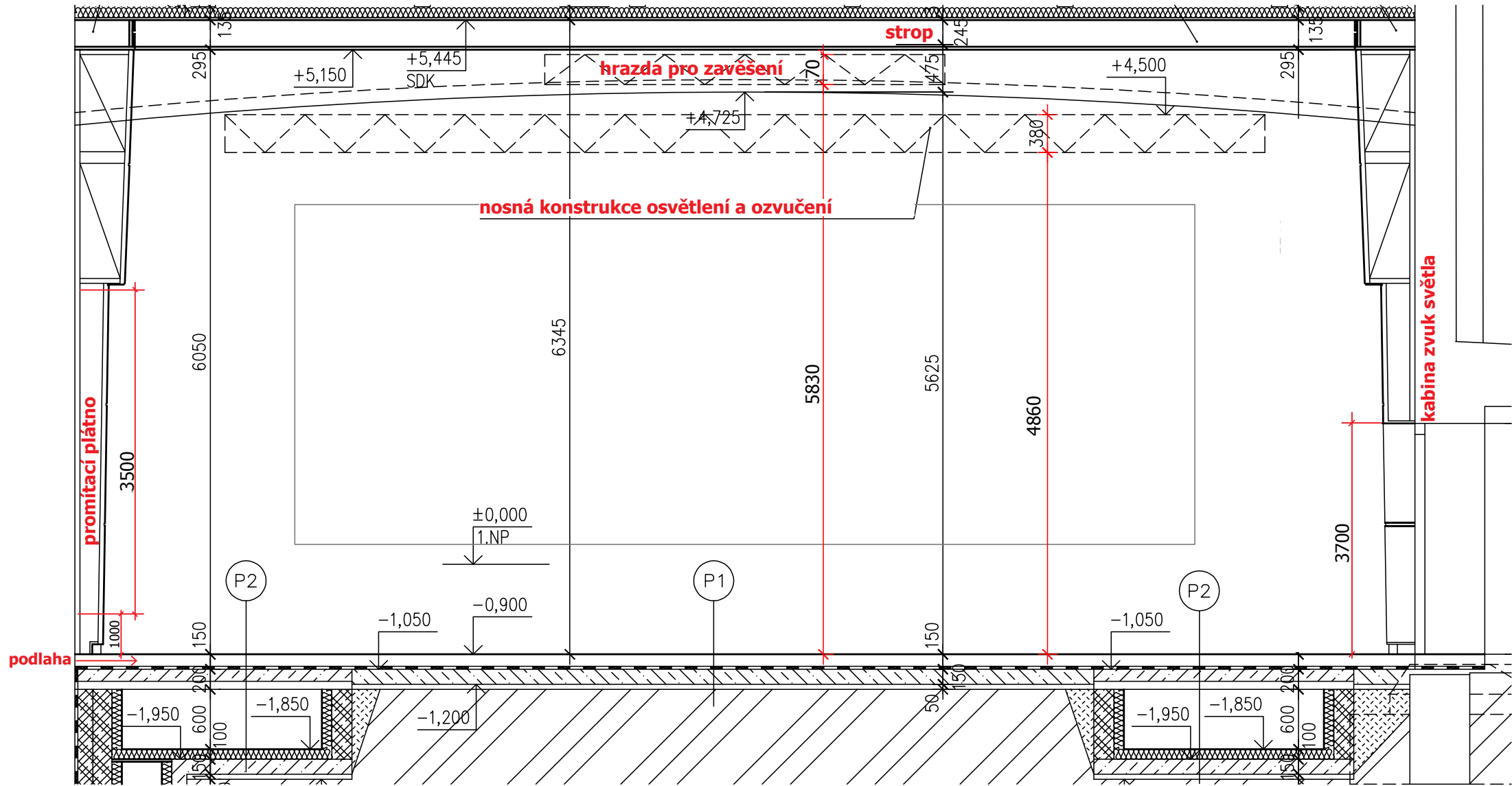
Řez sálem DIOD
